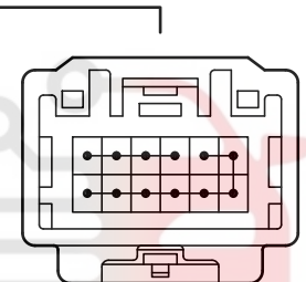
90980-12737
