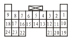
M23 ETACS A سفید
