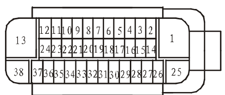
E04 ABS (ای.بی.اس)
