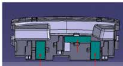
جایگاه تنظیم تشک‌ها هنگامی که زیر قاب بالابر در هستند
