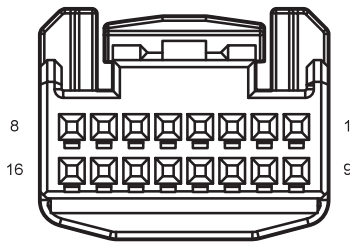
D05 Left Front Door Main Switch
