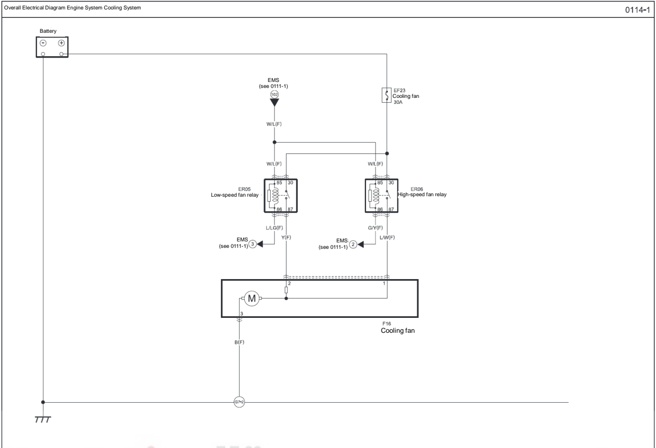
Cooling fan
