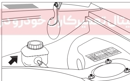
مخزن ترمز دو مداره تکلانتوس
