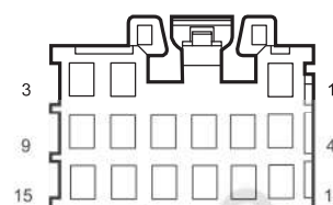
I_RLDB RL Door W.H. Connector Connecting Body W.H.
