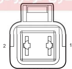
D23 RR Window Motor
