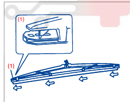
(۱) قفل انتها
