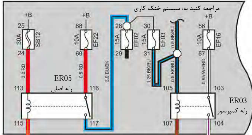
C01 فیوز محافظه موتور و جعبه رله
