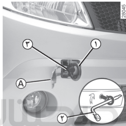
قلاب بکسل جلو ۳
