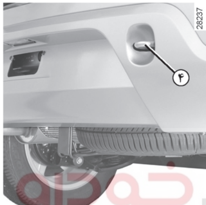
قلاب بکسل عقب ۴
